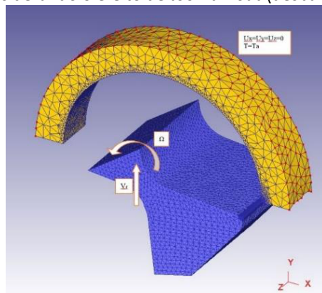
Figura 6. Simulação 3D considerando o efeito de tool run-out (desbalanceamento da ferramenta)
