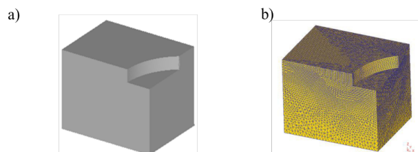
Figura 7. (a) Modelo CAD da peça e da ferramenta para microusinagem; (b) Malha FEM aplicada na simulação do processo de microusinagem
