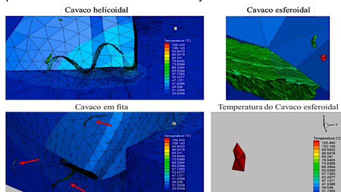
Figura 11. Tipos de cavacos formados na simulação do microfresamento do Inconel 718
