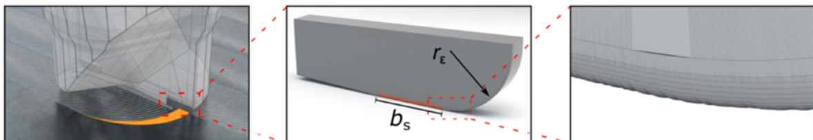
Figura 5. Modelagem do projeto da ferramenta e da aresta de corte para MRS
