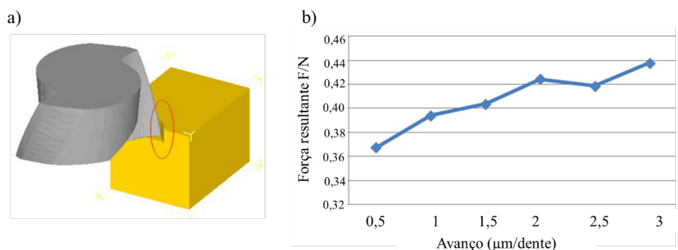
Figura 8. (a) Formação de cavacos em diferentes avanços por dente ( f_z ); (b) Variação da força de corte em função dos parâmetros de microusinagem
