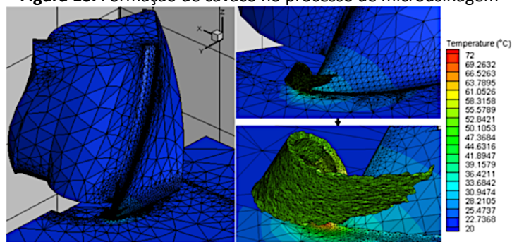
Figura 10. Formação de cavaco no processo de microusinagem
